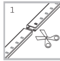
חיתוך חבל אור יעשה לפי הסימון בלבד ועם כלי מתאים
