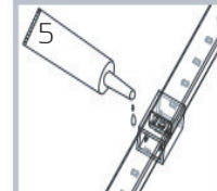
בזמן חיבור בין קצוות חבלי האור יש לשים סיליקון מבודד באזורי החיבור
