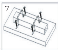
נתב וקבע את חבל האור בעזרת מפסניות יעודיות וברגים כמתואר
